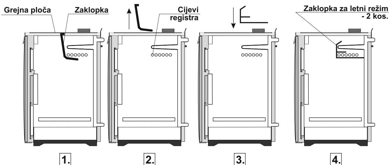
Slika 4. - Umetanje zaklopke za letni režim
